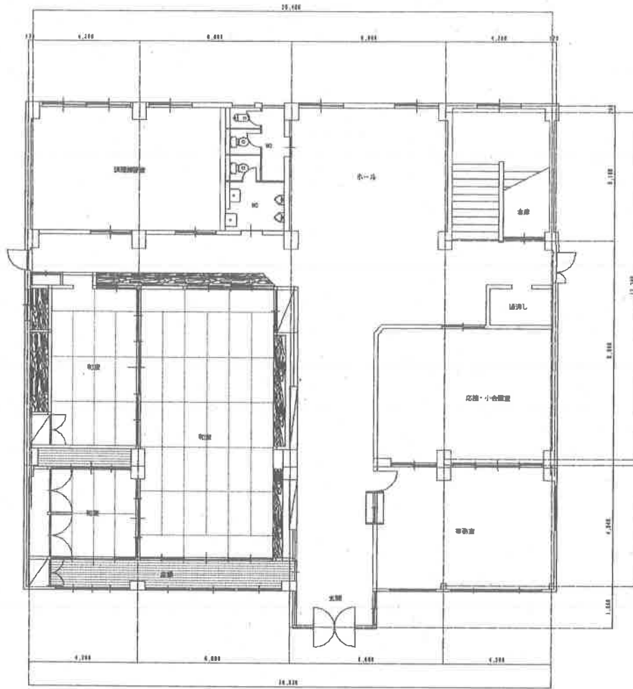
1階平面図
