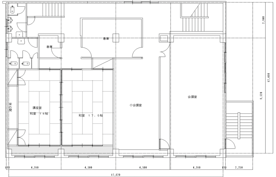
2階平面図
