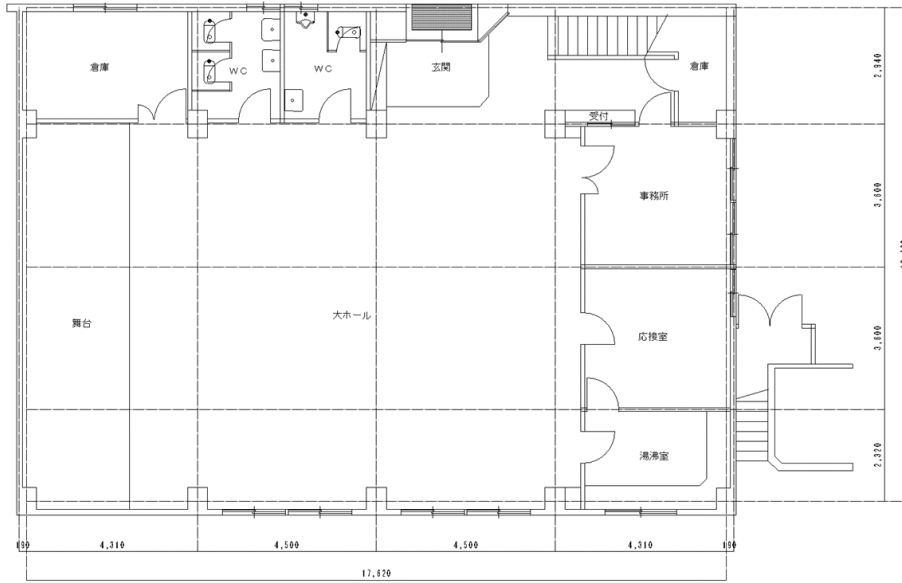
1階平面図
