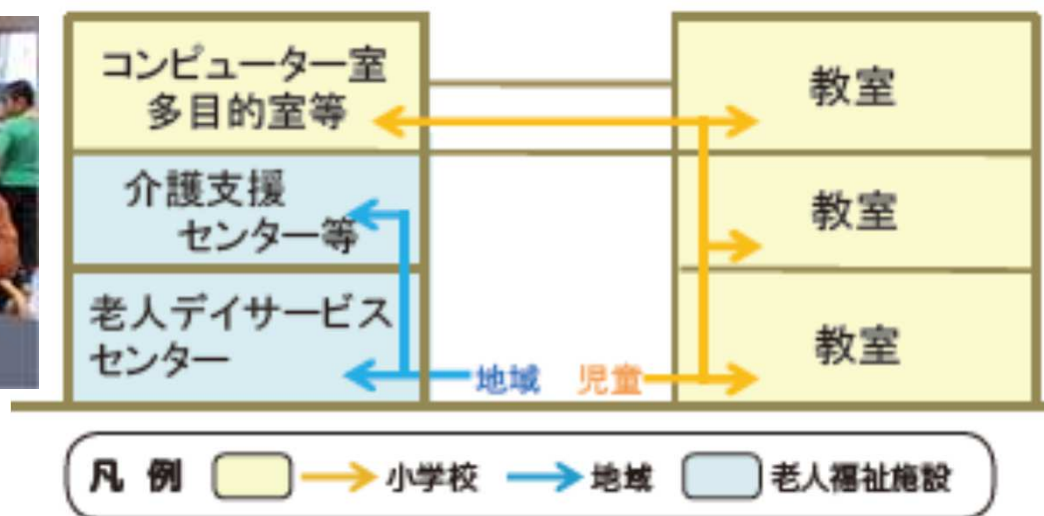
<立面図>
