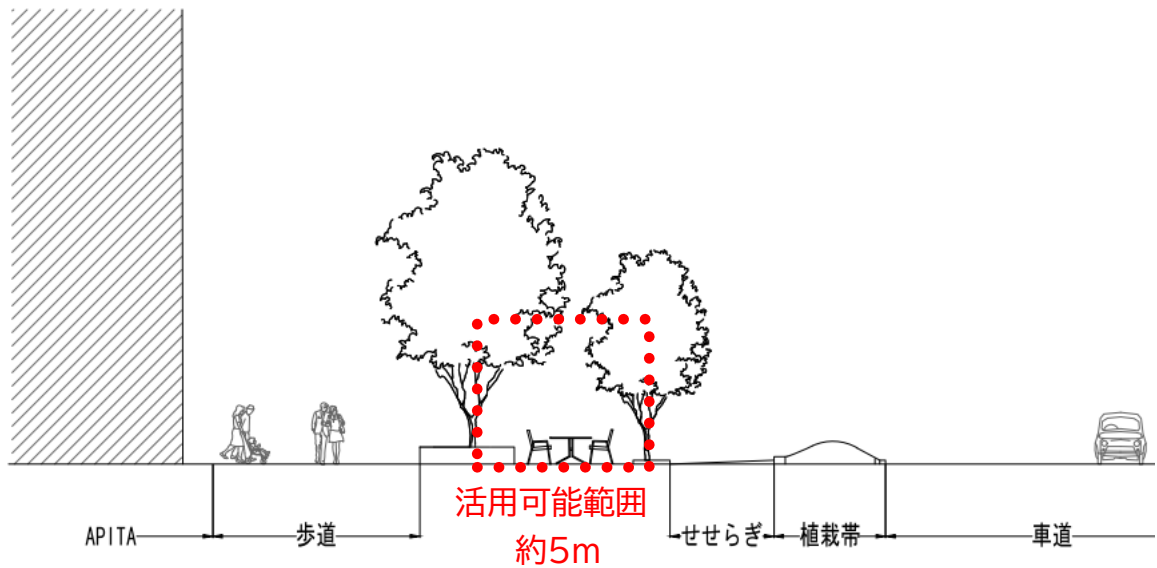
アピタ蒲郡店前横断面図
