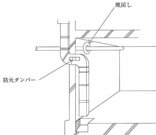
延焼のおそれのある外壁に設ける開口部の措置
