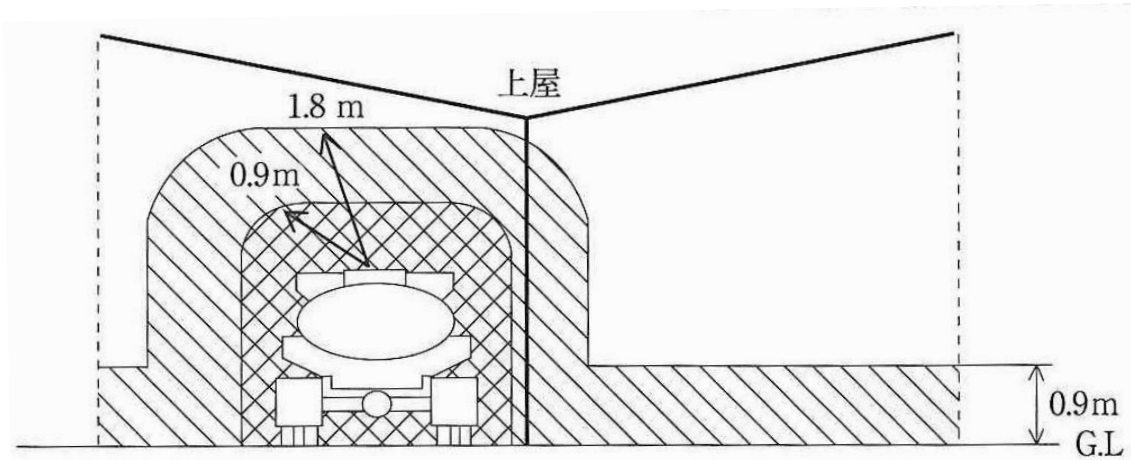
図 2 上屋を有するローリー積場
