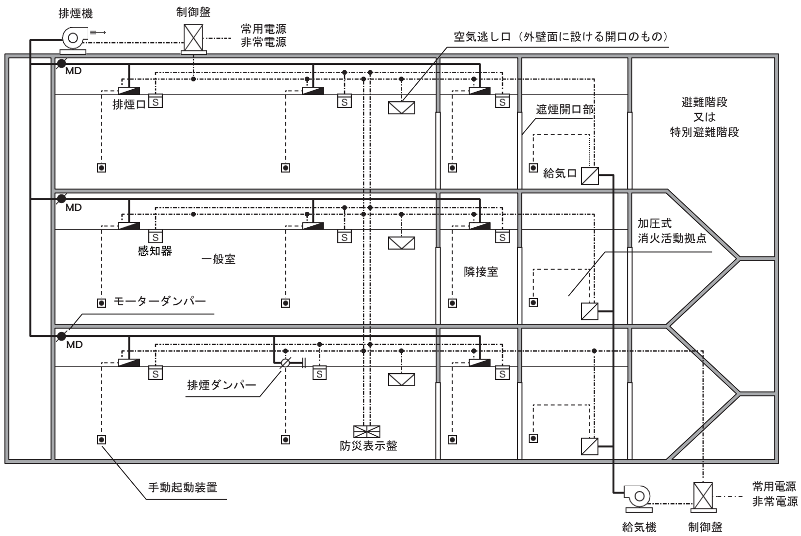
(1) 機械排煙方式 (第18の2-2図参照)
