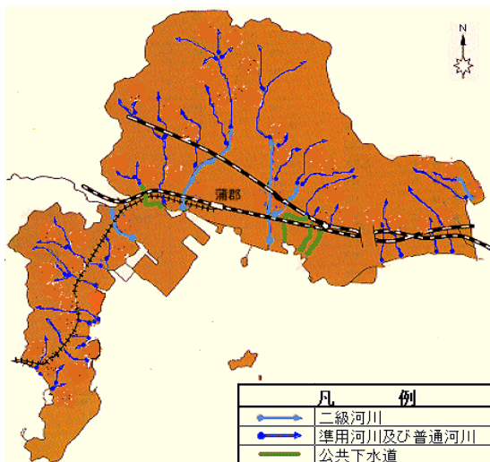
図 河川及び主な公共下水道雨水幹線
