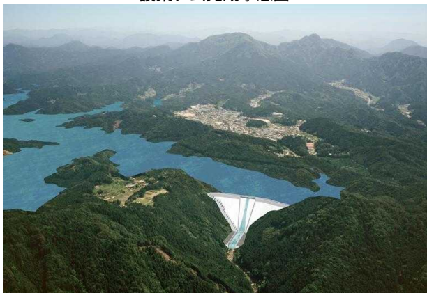
設楽ダム完成予想図
