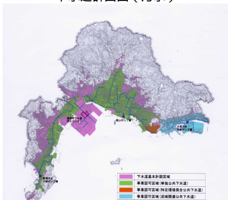
下水道計画図（汚水）
