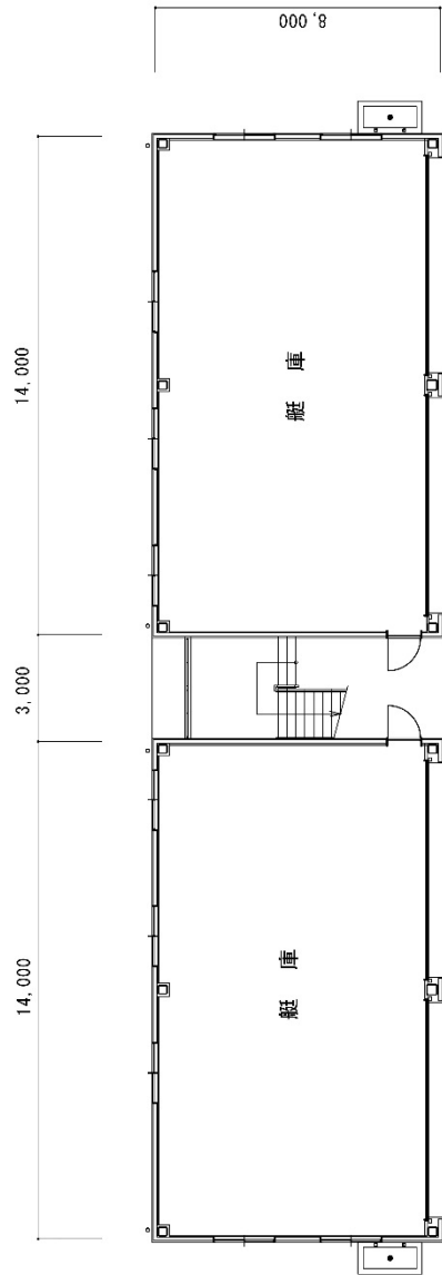
1 階 平 面 図
