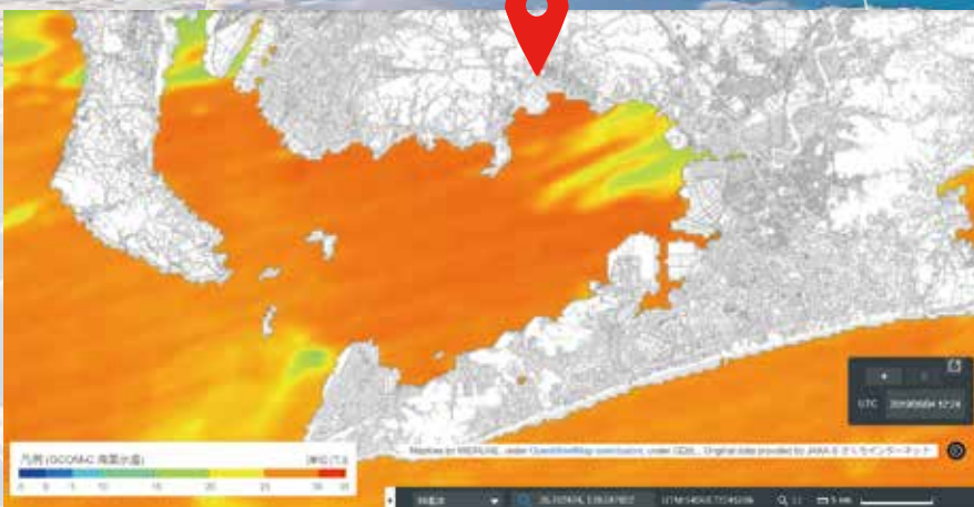
衛星画像でみる海面水温の様子 (河口付近の沿岸部等で温度が低くなっている様子が見える)
