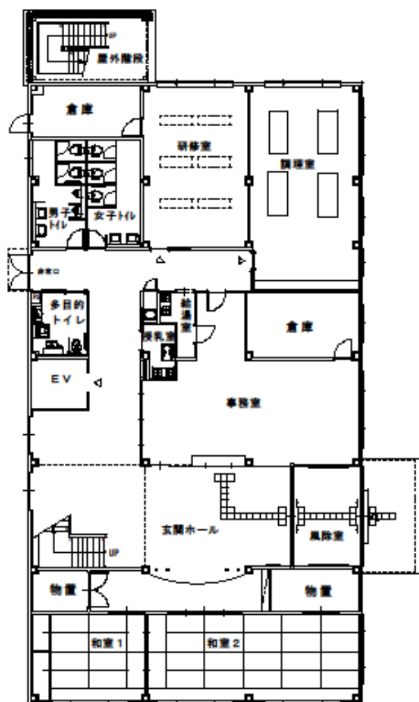
1 階
