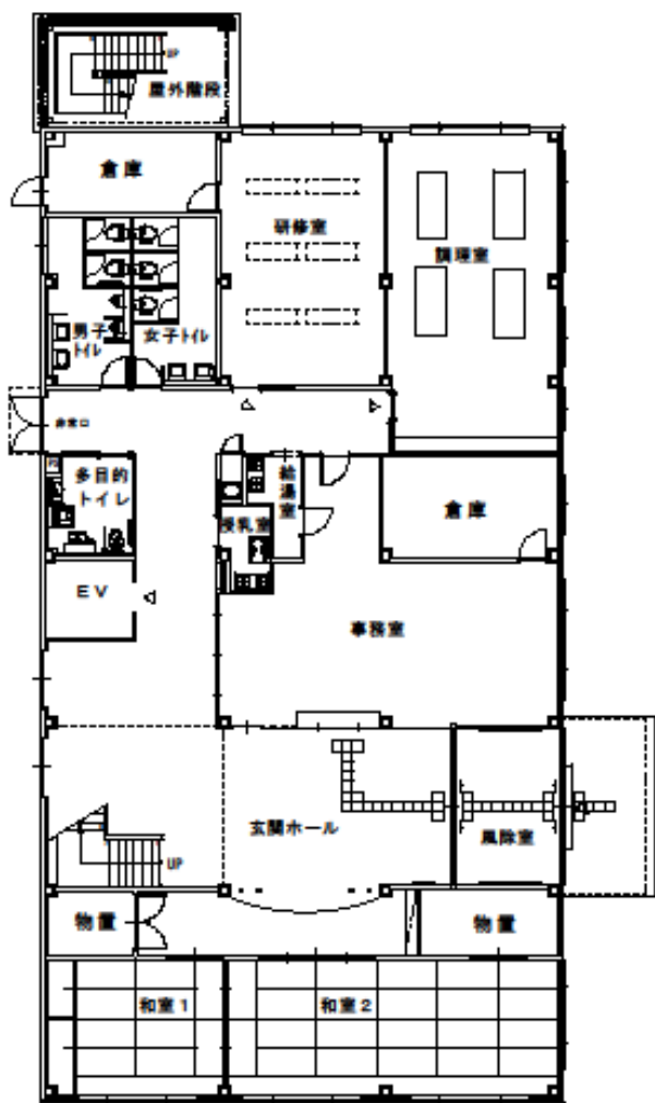
1 階
