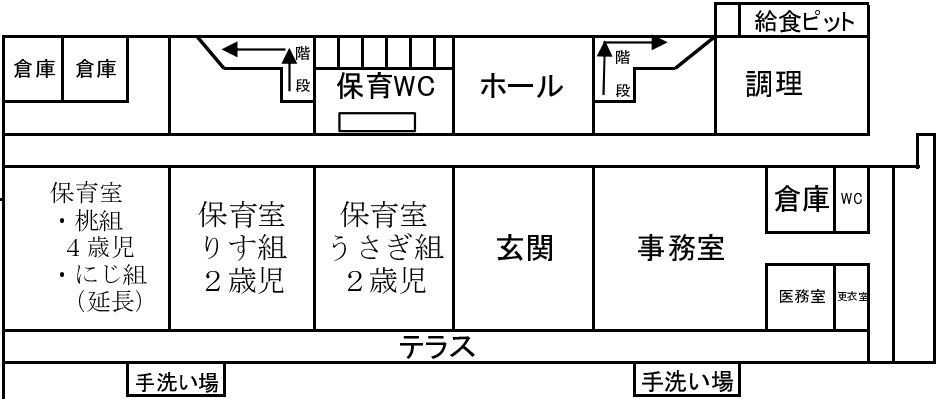
2階平面図
