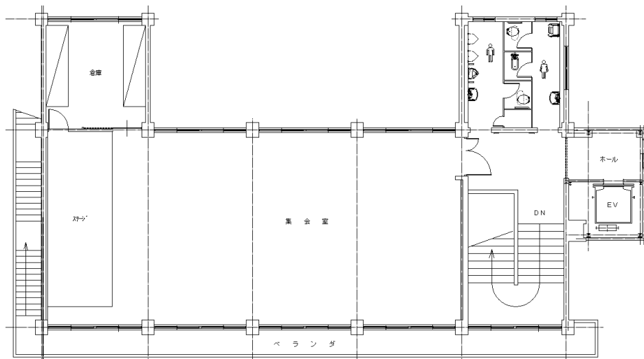
3階
