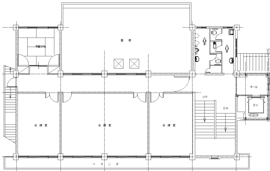
1階
