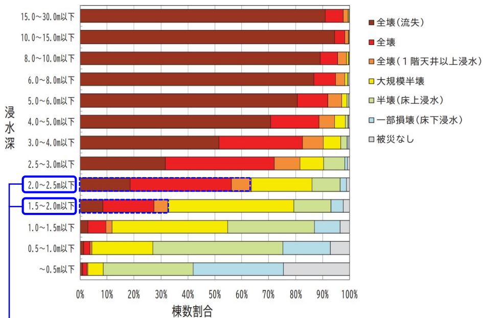
■ 浸水深に対する建物被害の割合
