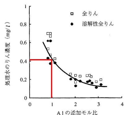
図 6-4 処理水のりん濃度と Al/P モル比の関係
