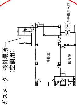
1階部分平面図
