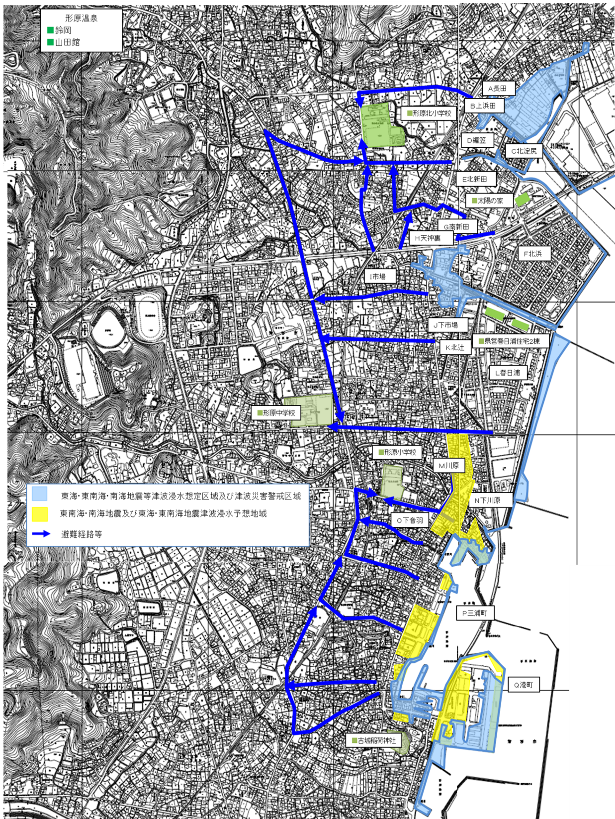
南海トラフ地震等の津波浸水想定区域等(形原町、金平町 図5)
