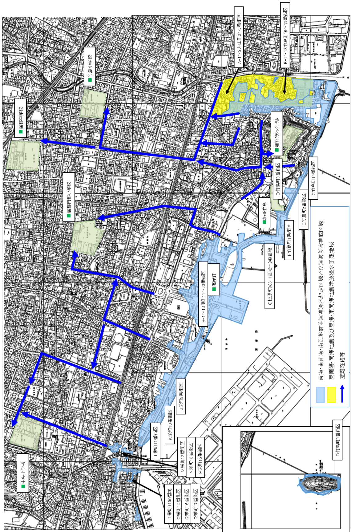
南海トラフ地震等の浸水想定区域等(丸山町、竹島町、松原町、港町、栄町 図3)
