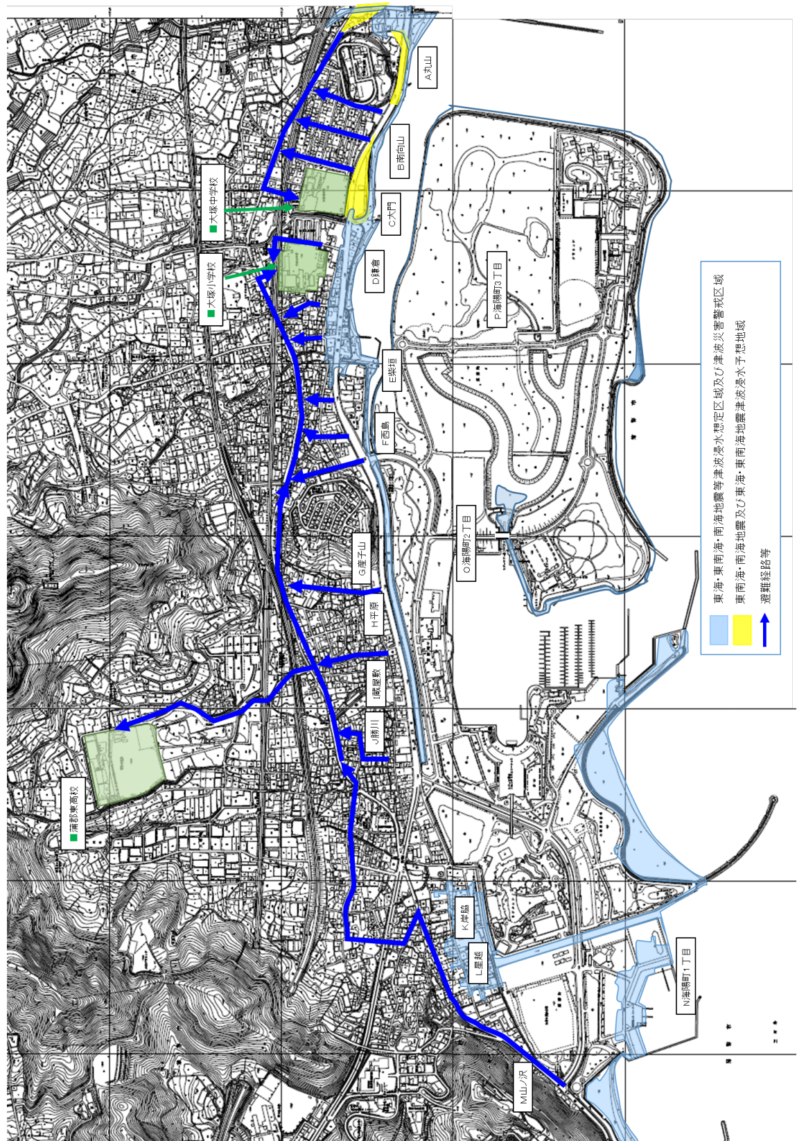
南海トラフ地震等の津波浸水想定区域等(大塚町、海陽町 図1)
