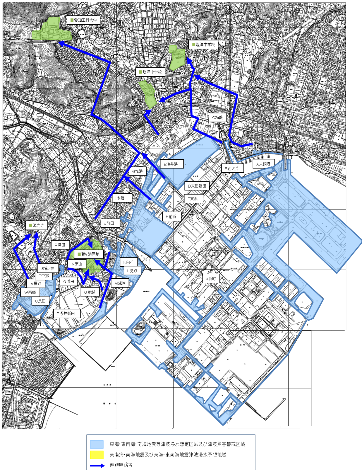
南海トラフ地震等の津波浸水想定区域等(浜町、竹谷町、拾石町、鹿島町 図4)
