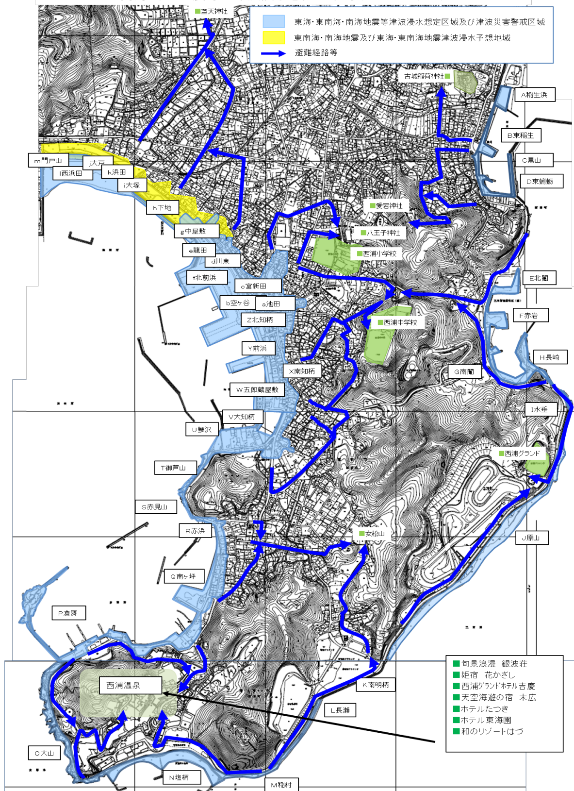
南海トラフ地震等の津波浸水想定区域等(西浦町 図6)
